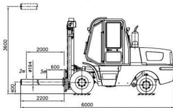
Стрела крановая 451A.52.00.000-Б
