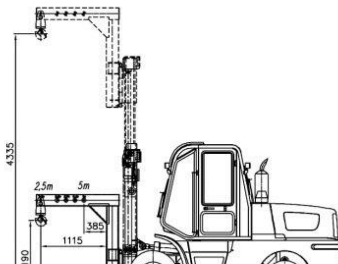
Стрела крановая 451A.52.00.000-Б
